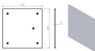
EMBASE LÉGÈRE CARRÉE 35X35 ALU EM259
