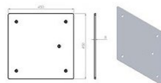
EMBASE LÉGÈRE CARRÉE 30*30CM ALU EM259
