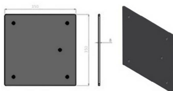
EMBASE LÉGÈRE CARRÉE 30*30 NOIRE EM259
